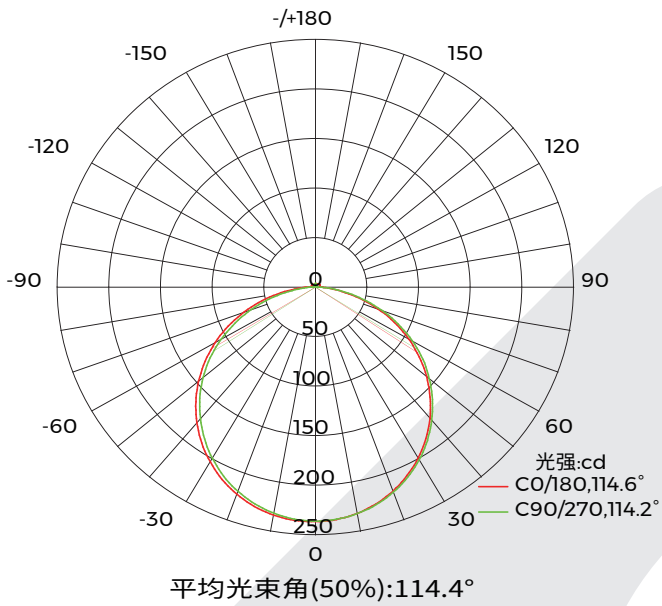
配光曲线
